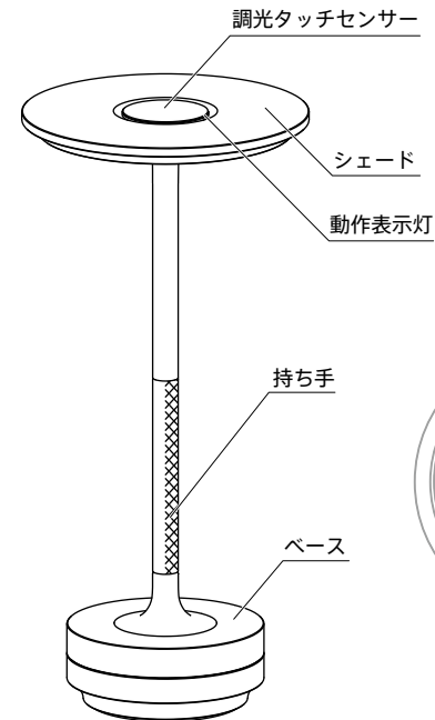
本体
